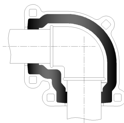
图 23 钢管弯头哈夫节施工示意图
