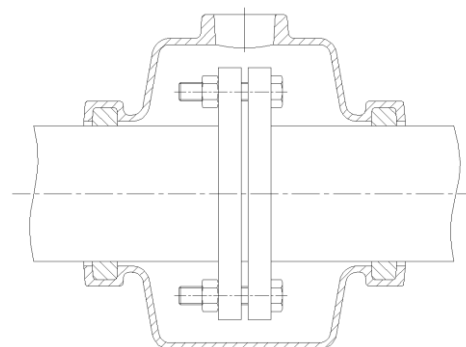
图 6 法兰哈夫节施工示意图
