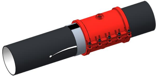
图 39 固定连接器，安装哈夫节
