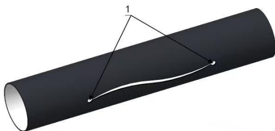
1-应力释放孔
