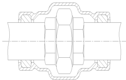
图 20 钢管活接哈夫节施工示意图
