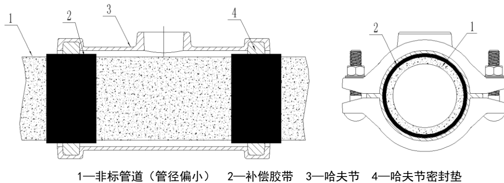
图 36 非标偏小管道的施工作业
