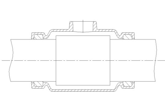
图 9 塑料管承插哈夫节施工示意图
