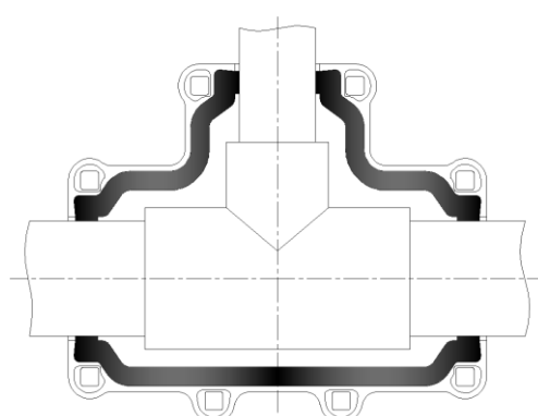
图 12 塑料管异径三通哈夫节施工示意图
