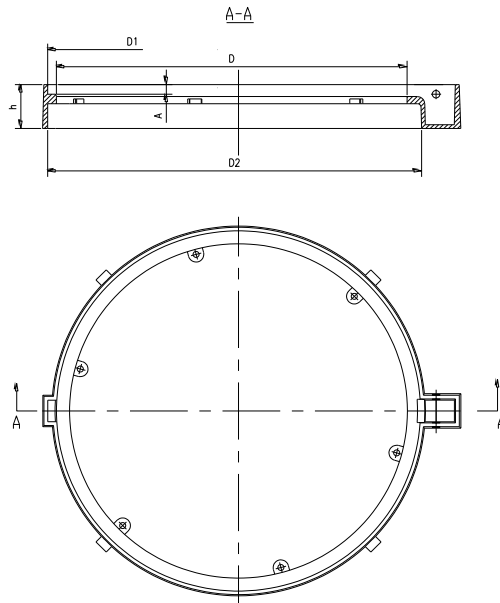
图 E. 25 简易井座结构尺寸示意图
