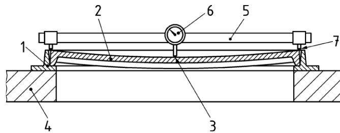
1-井座或井(箅)圈 2-井盖或箅子 3-几何中心 4-试验机的底座 5-测量仪器支架 6-测量仪器 7-测量仪器支架底座
