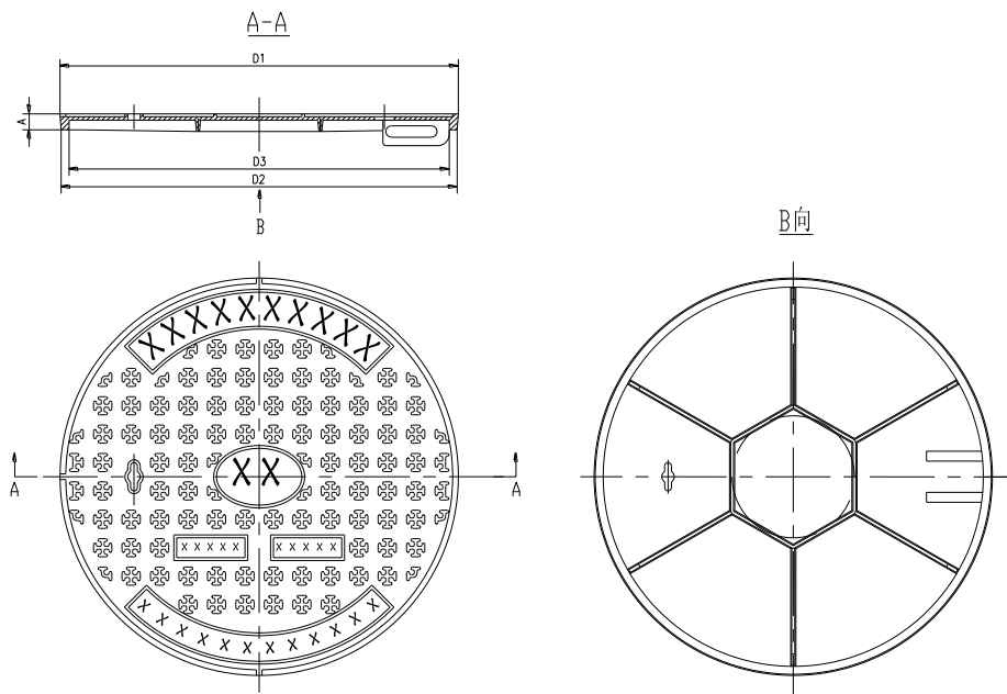
图 E.1 A 级和 B 级井盖结构尺寸示意图
