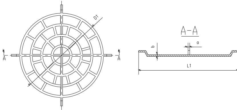
图 E.8 防坠落格栅结构尺寸示意图
