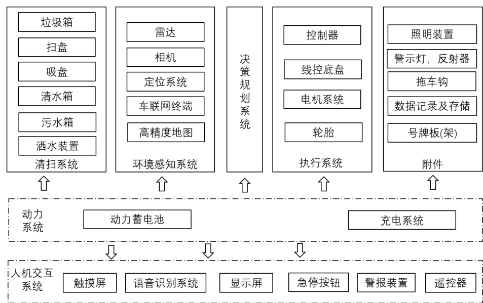
图1 无人驾驶清扫装备结构示意图
