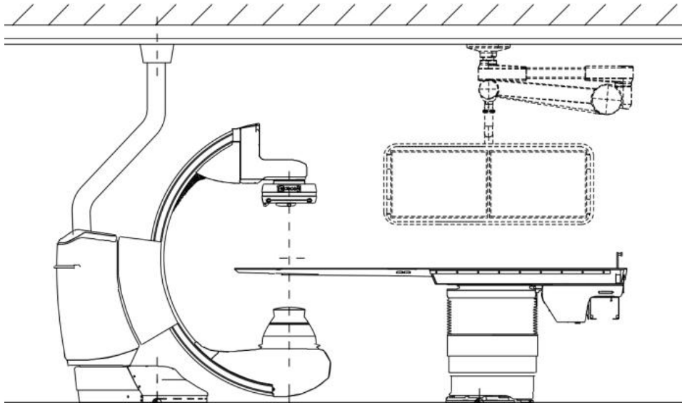
图A-2 落地式DSA图示
