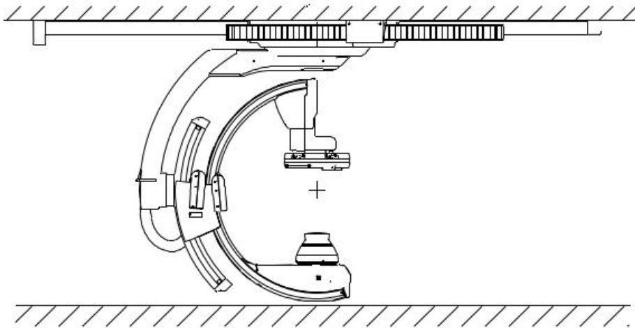
图A-1 悬吊式DSA图示
