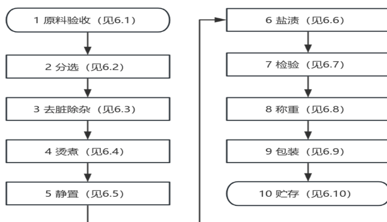
图1 盐渍海参加工工艺流程图
