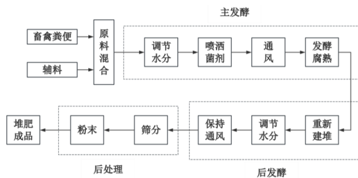
图 2 条垛式免翻堆堆肥工艺流程示意图
