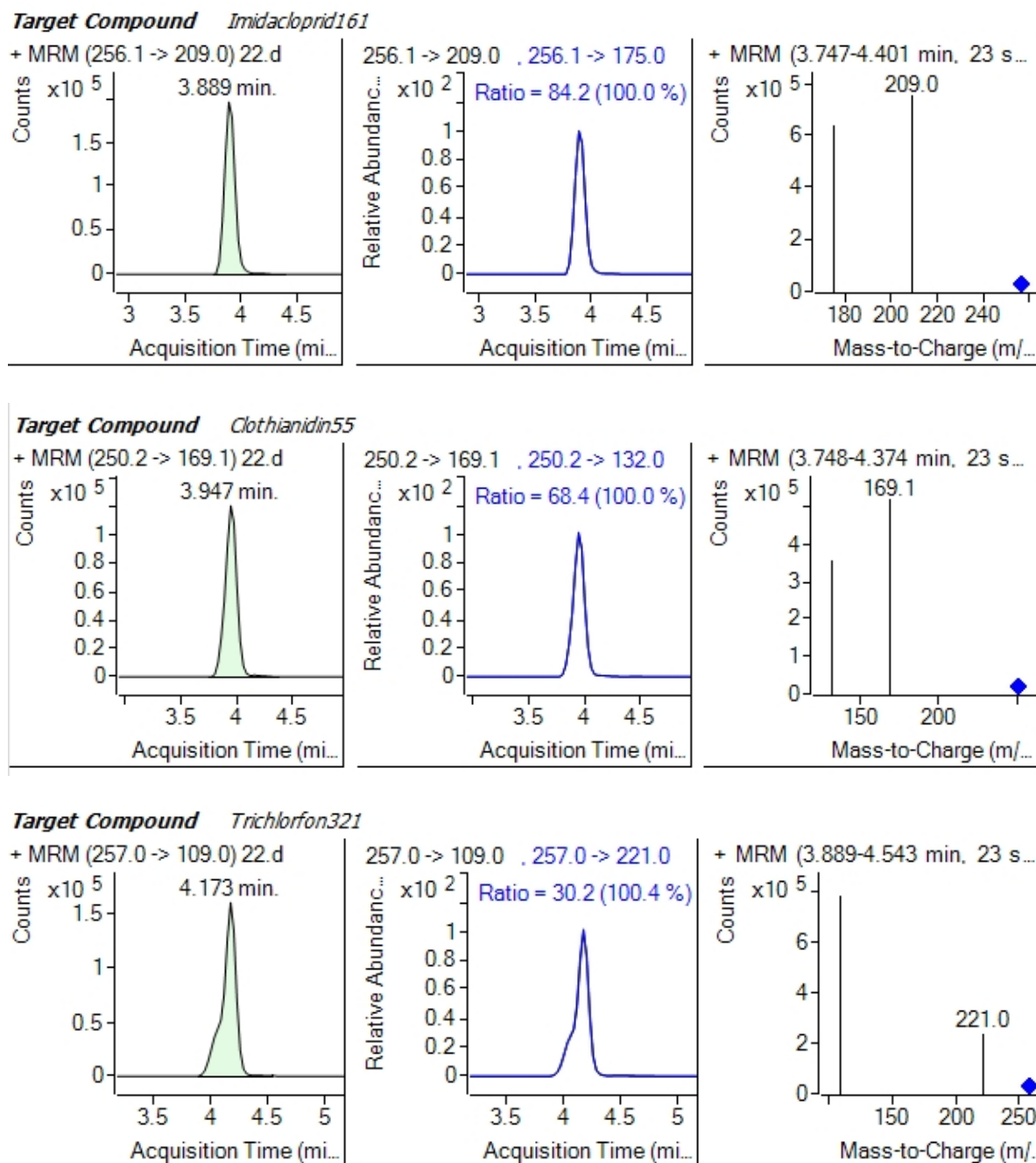
图 C.1 各种农药的多反应监测 (MRM) 色谱图
