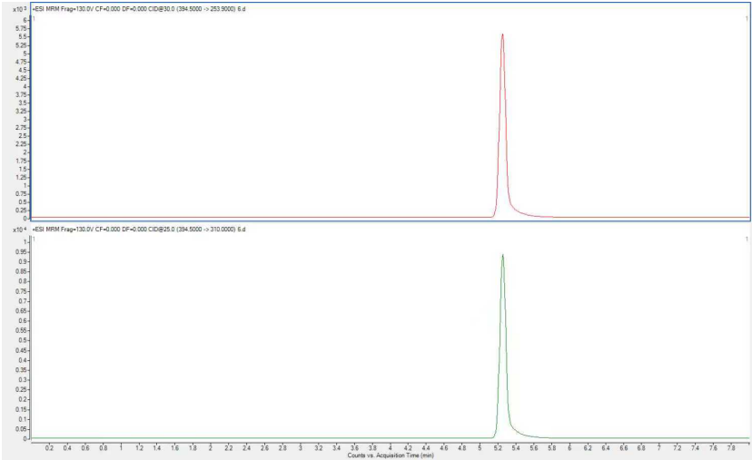
图 C.1 脲吡喃酯的多反应监测（MRM）典型色谱图
