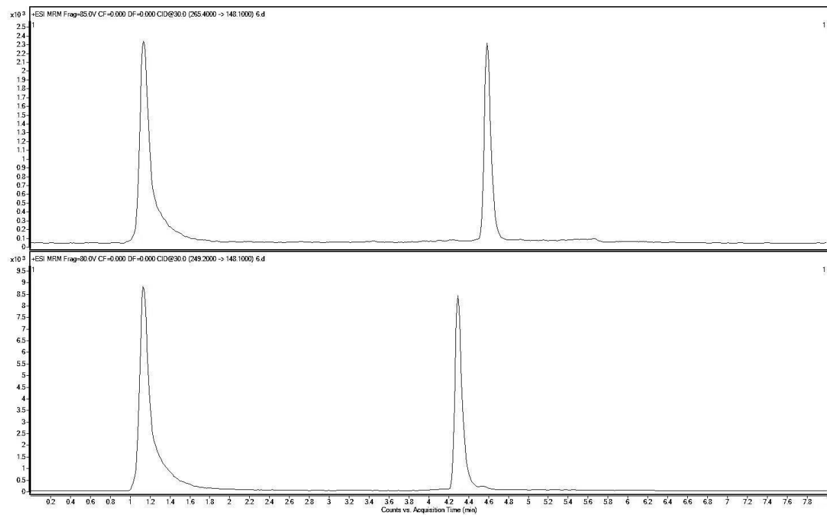
图 C.1 苦参碱和氧化苦参碱的多反应监测（MRM）典型色谱图
