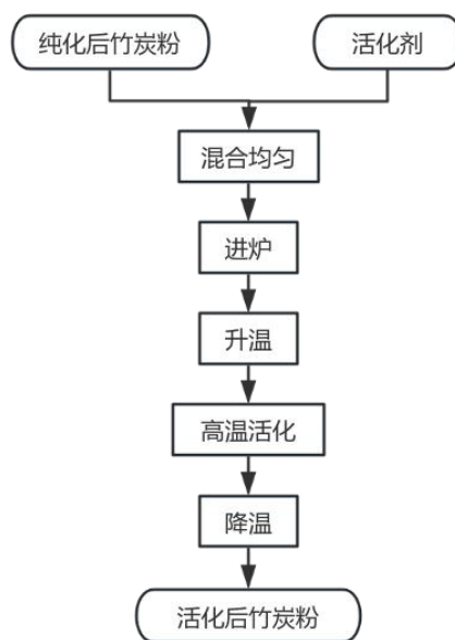
图5 表面处理流程图
