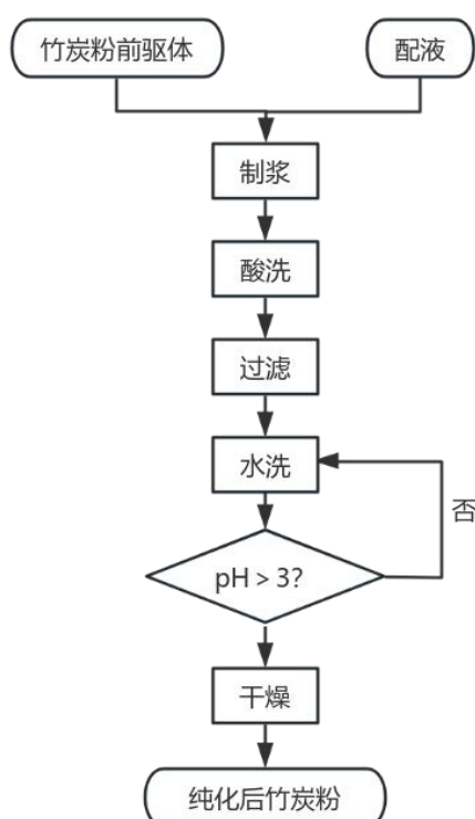
图 4 酸洗纯化流程图
