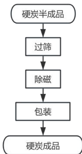
图7 成品工艺流程图
