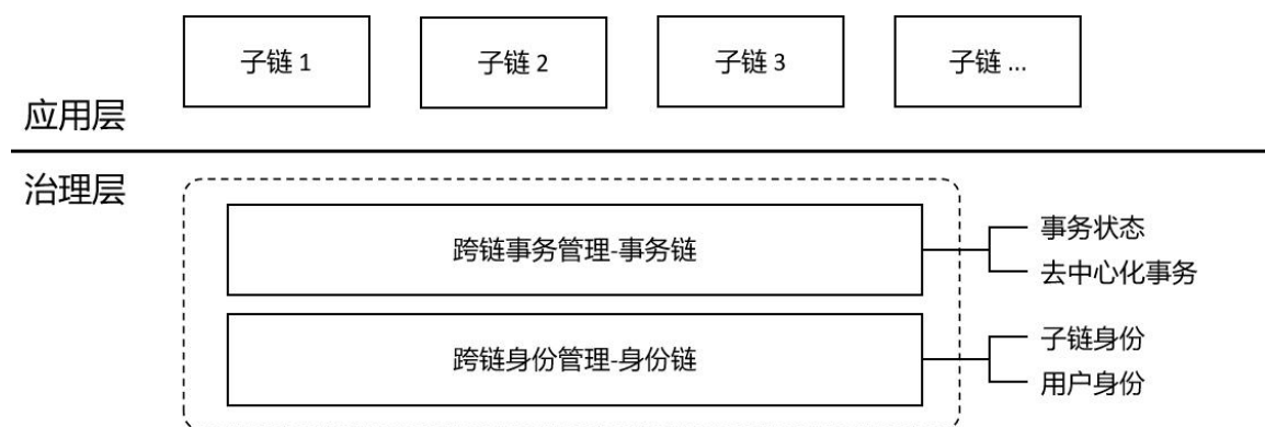
图 1 政务区块链跨链系统架构
