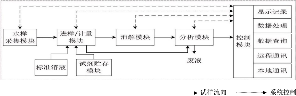
图1 自动在线监测仪器的基本组成单元
