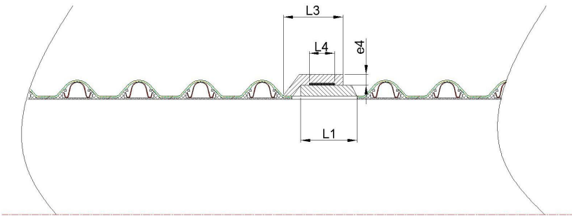
图 A. 9 承插式橡胶密封圈连接
