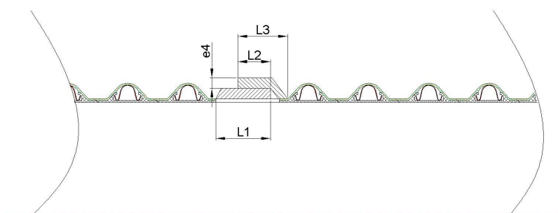
图 A.8 锥形承插式电熔连接
