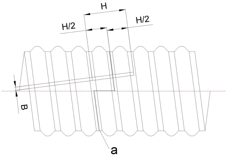
图 E. 1 焊缝或熔缝的拉伸强度制备试样的尺寸
