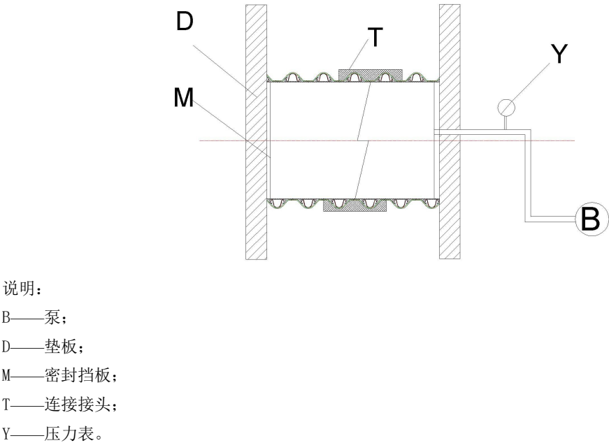
图 D.1 水压密封试验装置示意图
