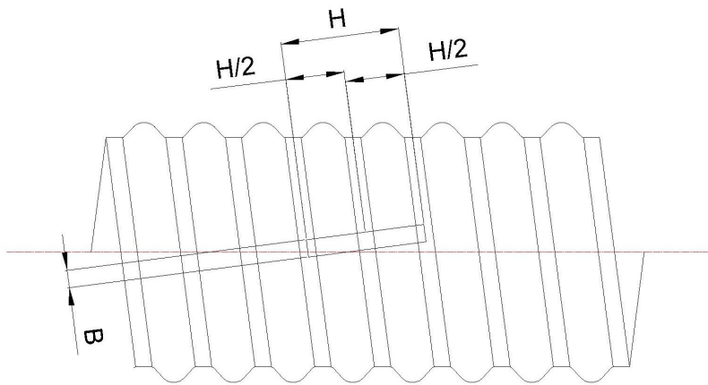
图 C.2 层压壁的拉伸强度制备试样的位置
