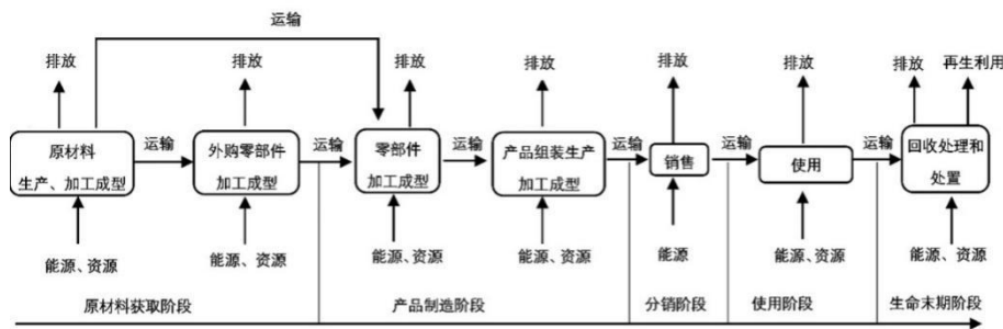
图1 电吹风产品碳足迹评价的系统边界示例
