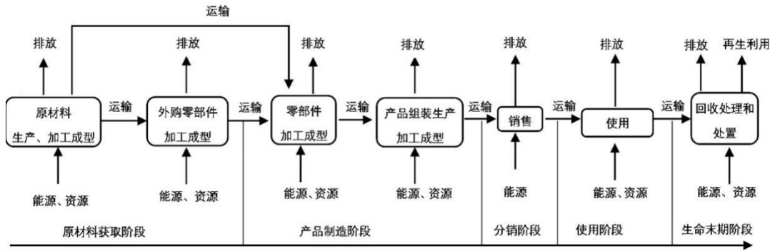
图1 室内加热器产品碳足迹量化的系统边界示例
