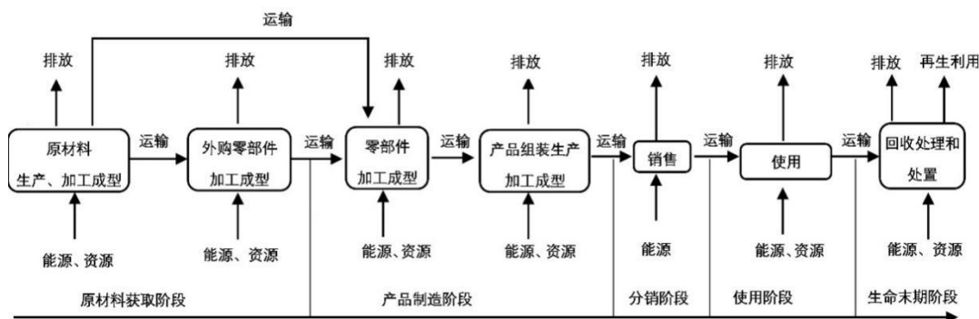
图1 电风扇产品碳足迹量化的系统边界示例
