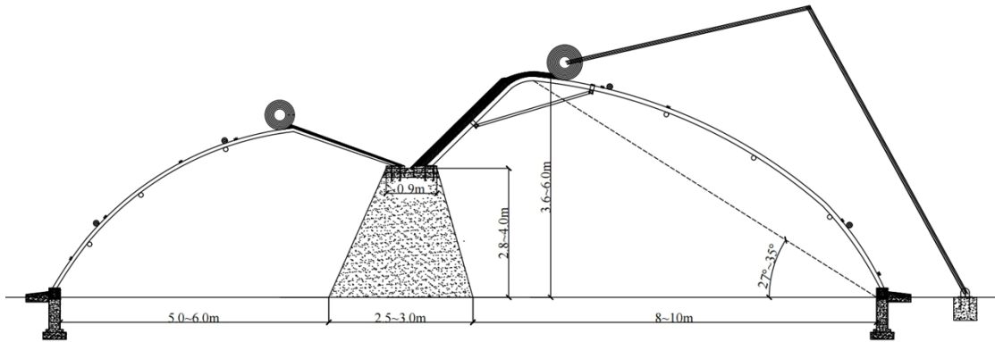
老旧厚土墙日光温室双连跨改造剖面示意图
