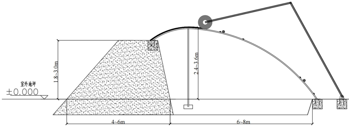
老旧厚土墙日光温室双连跨改造剖面示意图
