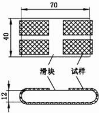
图 A.3 摩擦因数试验试样固定示意图
