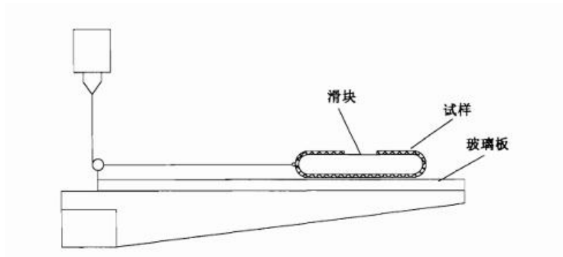
图 A. 4 摩擦因数装置示意图
