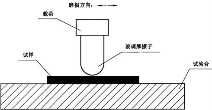
图 A.1 磨损检测装置图
