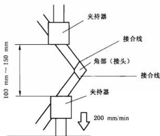
图1 角部结合力(接头扯断力)试验示意图
