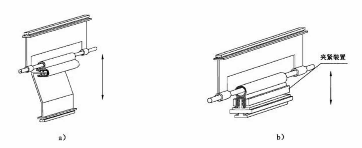
图 A.5 密实胶与海绵胶扯断力试验装置示意图
