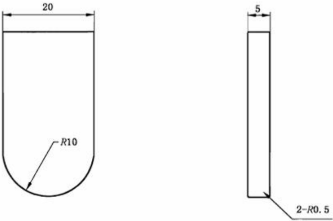
图 A.2 玻璃摩擦子示意图
