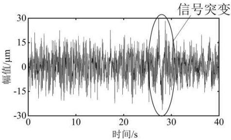
图 B.2 含较强噪声振动波形
