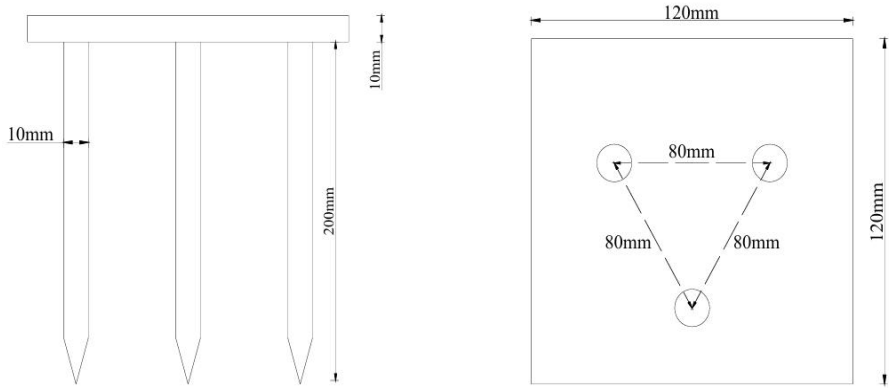
图 2 专用底座参考尺寸
