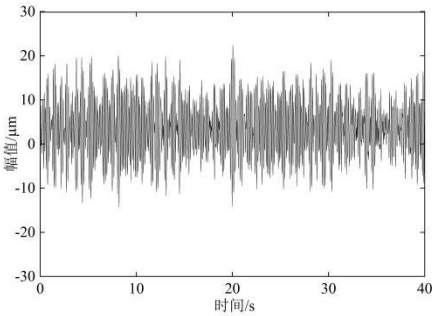
图 B.3 零点漂移振动信号图
