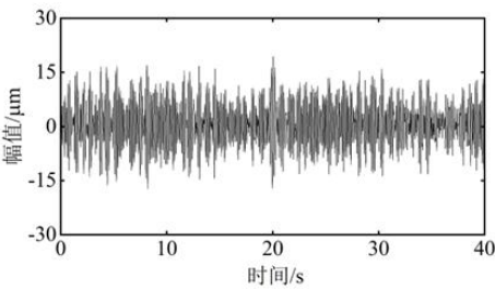
图 B.1 正常平稳随机振动波形
