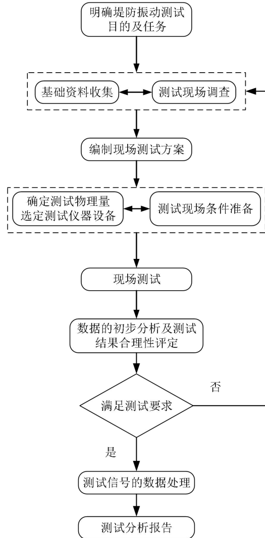
图 A. 1 堤防振动测试流程图
