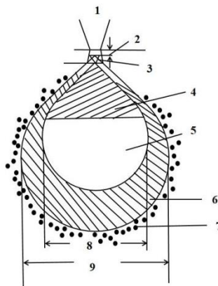
1.入射电子束 2.俄歇电子 3.二次电子 4.背散射电子 5.特征 X 射线 6.连续 X 射线 7.由连续和特征 X 射线激发的二次荧光 8.背散射电子的空间分辨率 9. X 射线的分辨率
