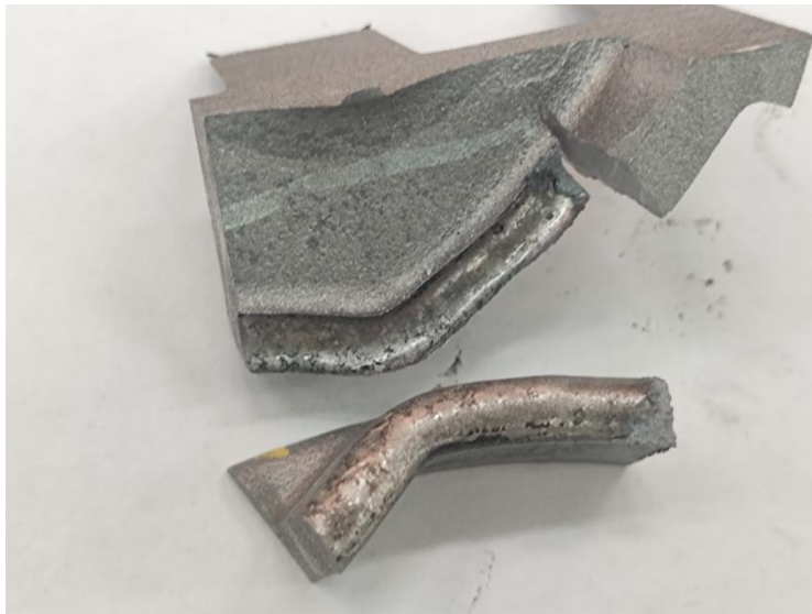
图16 排气管 QTRS4Mo1 薄管壁处 冷隔缺陷形貌
