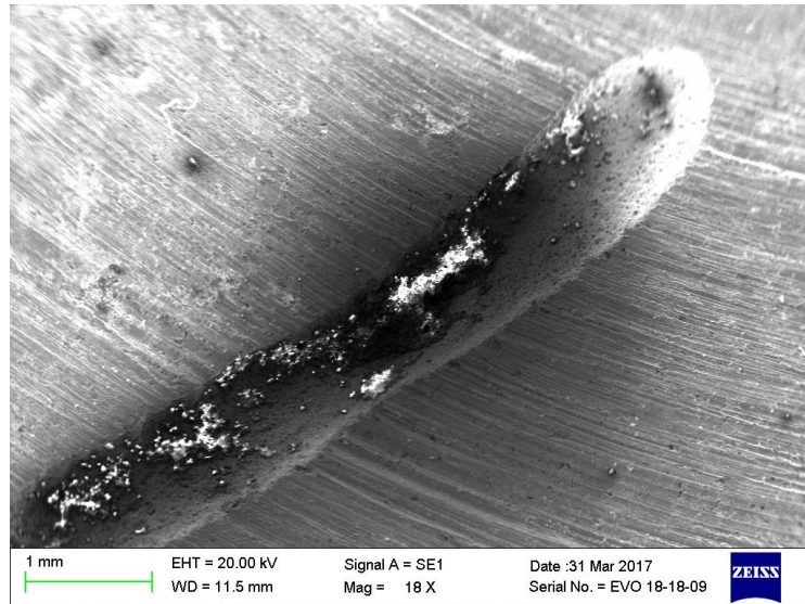
图 13 缸盖 HT250 铸造顶部 过滤网破损 夹杂物缺陷形貌
