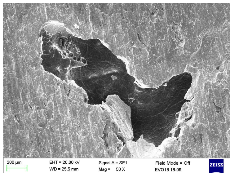
图9 机体 RuT450 副油道处气孔缺陷微观形貌
