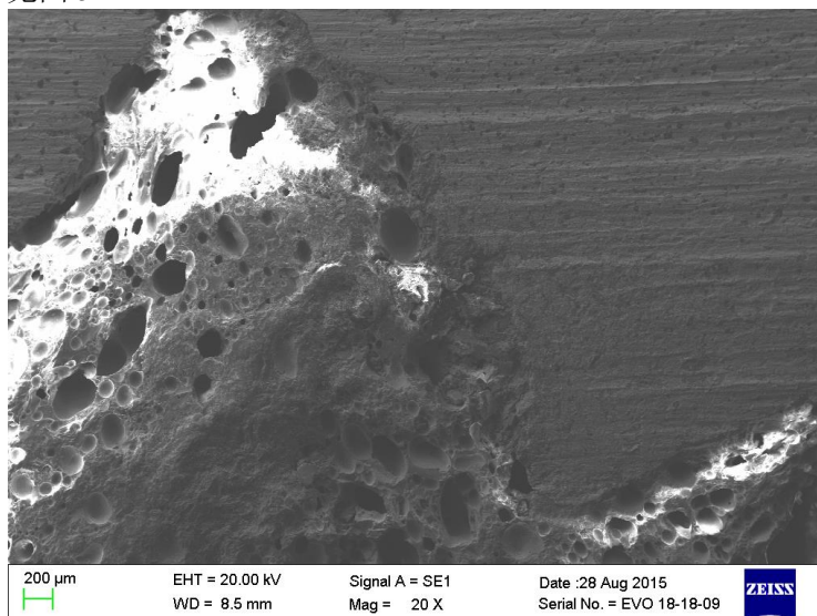
图 3 缸盖 RuT350 铸件顶部夹渣缺陷形貌
