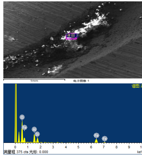
图 15 缸盖 HT250 铸造顶部 过滤网破损 夹杂物电镜能谱分析结果
