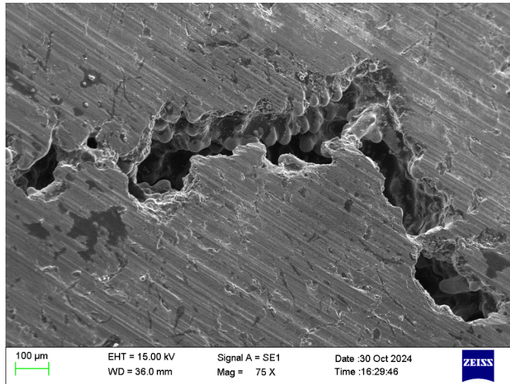
图 21 缸盖 HT300 阀座加工面 氮气孔缺陷形貌
