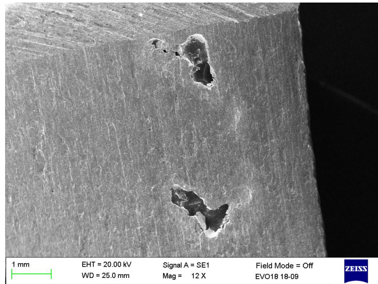
图8 机体 RuT450 副油道处气孔缺陷形貌
