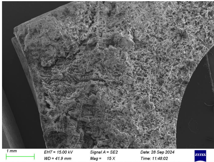
图 6 机体 HT250 主螺栓孔处 缩松缺陷形貌
