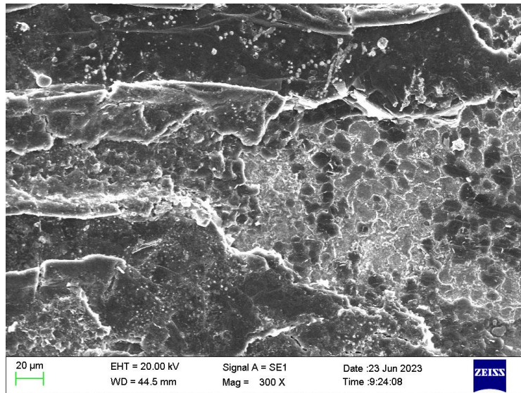
图17 排气管 QTRSi4Mo1 薄管壁处 冷隔缺陷微观形貌
