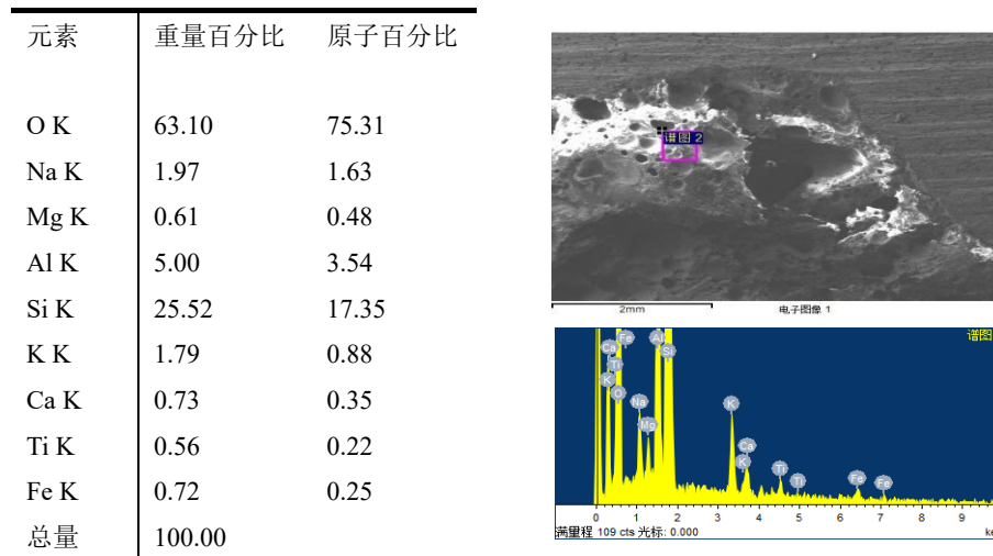
图5 缸盖 RuT350 铸件顶部夹渣处电镜能谱分析结果
