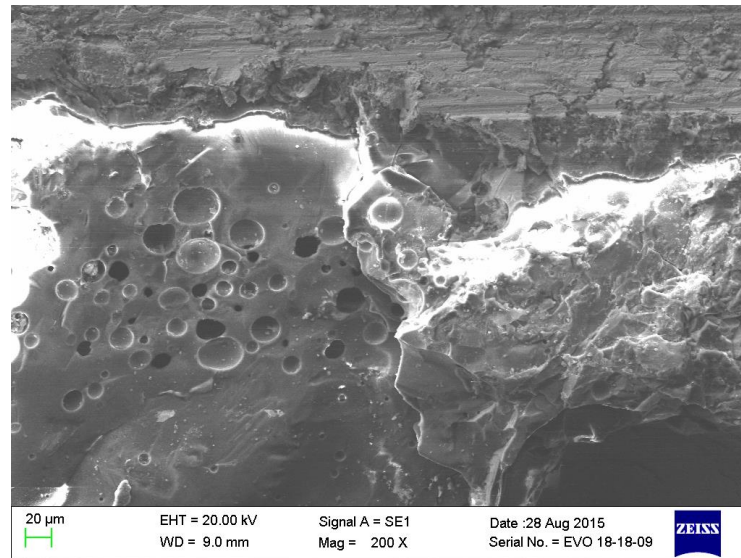
图4 缸盖 RuT350 铸件顶部夹渣缺陷微观形貌
