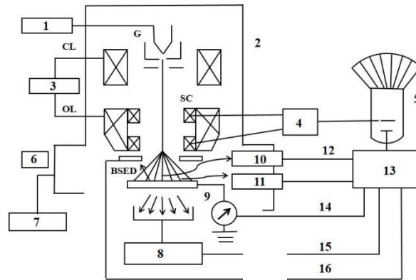
1.电子枪电源 2.镜筒 3.透镜电源 4.同步扫描发生器 5.荧屏 6.样品室 7.真空系统 8.透射电子探测器 9.样品 10.E-T 探测器 11.荧光探测器 12.二次电子 13.视频放大器 14.吸收电子 15.透射电子 16.背散射电子
