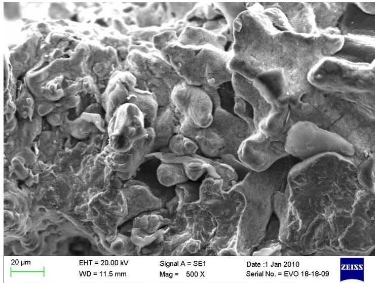
图 19 机体 HT250 底平面 热裂缺陷微观形貌
