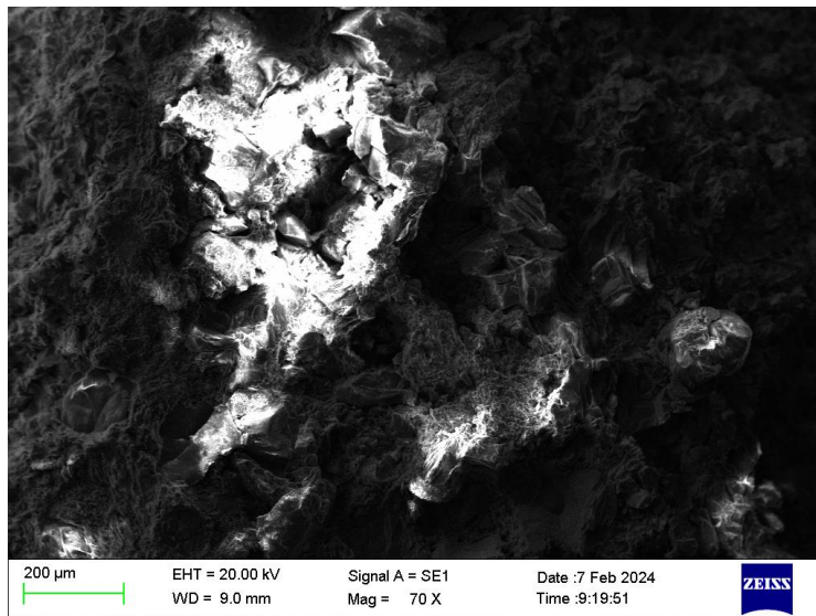
图 11 机体 HT250 底平面 砂眼缺陷形貌
