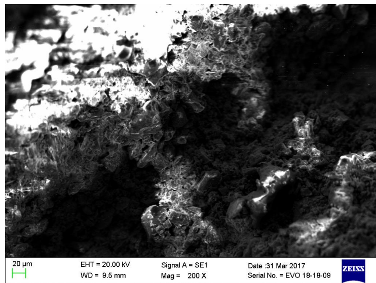
图 14 缸盖 HT250 铸造顶部 过滤网破损 夹杂物缺陷形貌
