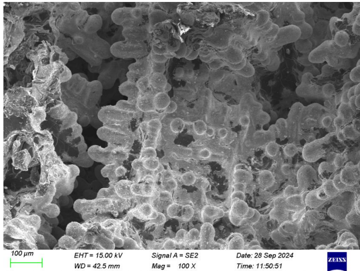
图 7 机体 HT250 主螺栓孔处 缩松缺陷微观形貌
