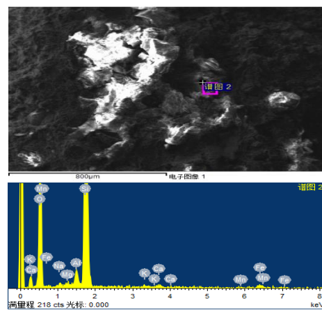
图12 机体 HT250 底平面 砂眼电镜能谱分析结果
