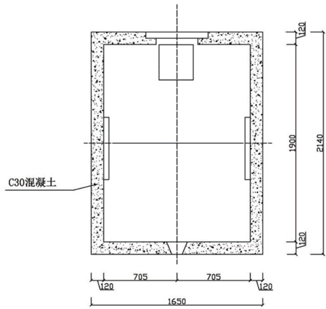
1960*1410*1900 (B-立面图)
