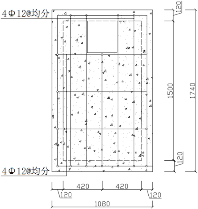
1450*840*1500 (B-立面图配筋图)
