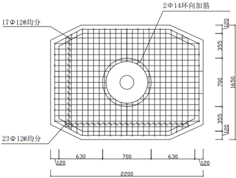
1960*1410*1900上覆盖配筋图
