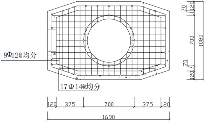
1450*840*1500上覆盖配筋图
