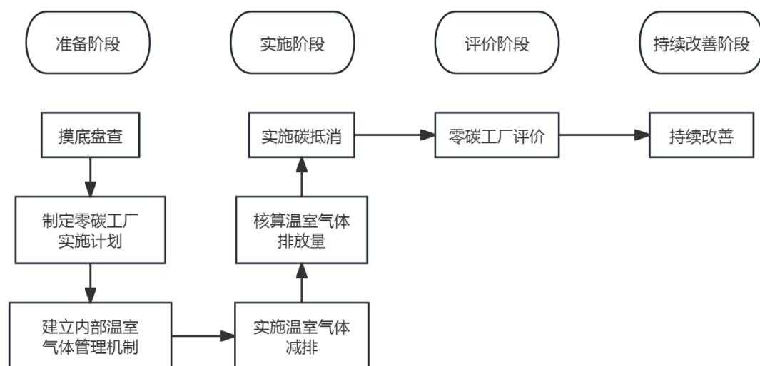
图1 零碳工厂实施流程图
