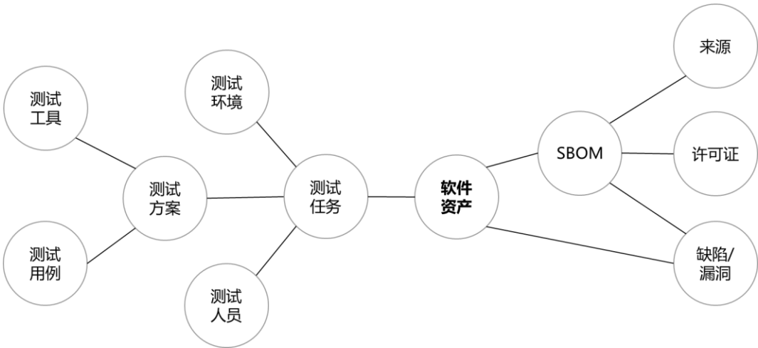
图 2 以资产为核心的测试要素关联关系
