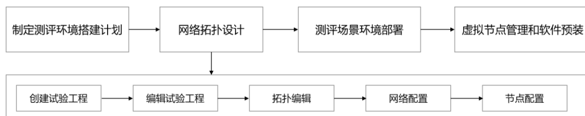
图 3 测试环境搭建流程
