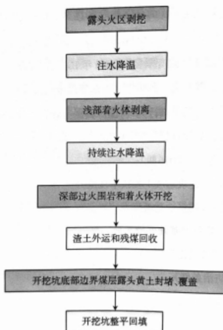
图 1 火区治理工艺流程图
