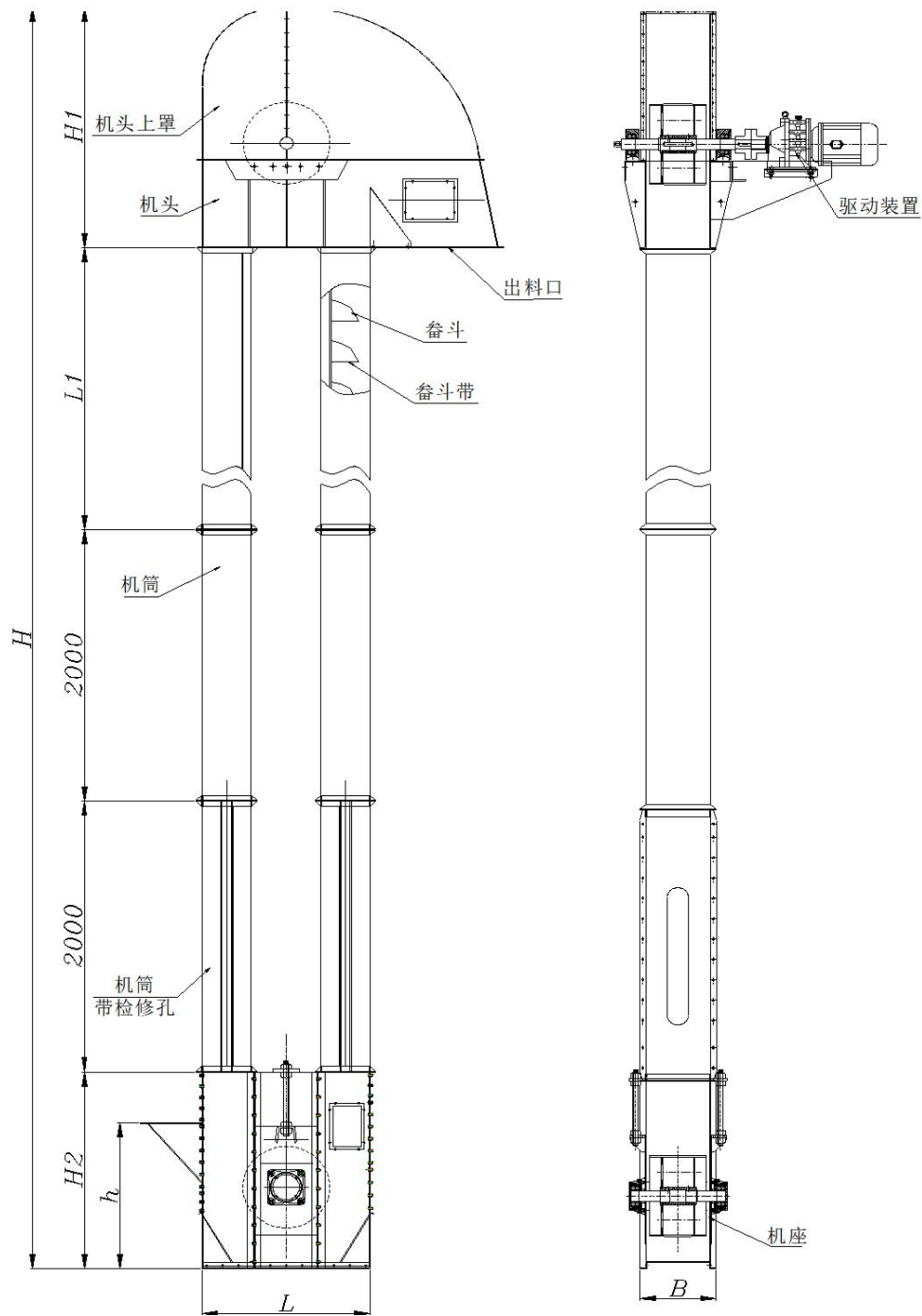
图 1 原粮慢速提升机结构示意图
