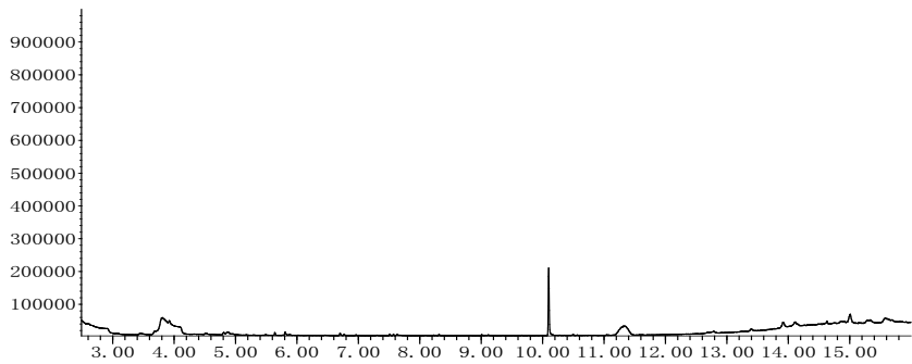
图 B.1 1,6-二氧杂环十二烷-7,12-二酮标准工作溶液总离子流色谱图
