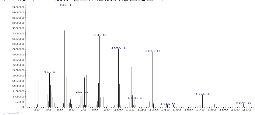
图 B.2 1,6-二氧杂环十二烷-7,12-二酮标准工作溶液质谱图
