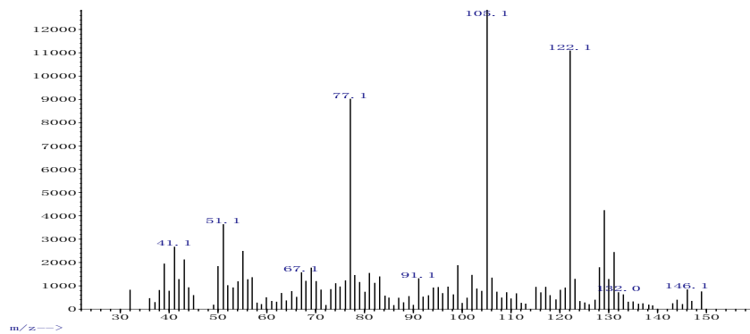
图 B.3 苯甲酸标准工作溶液质谱图
