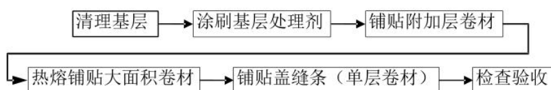
图3 弹性体改性沥青防水卷材施工工艺流程
