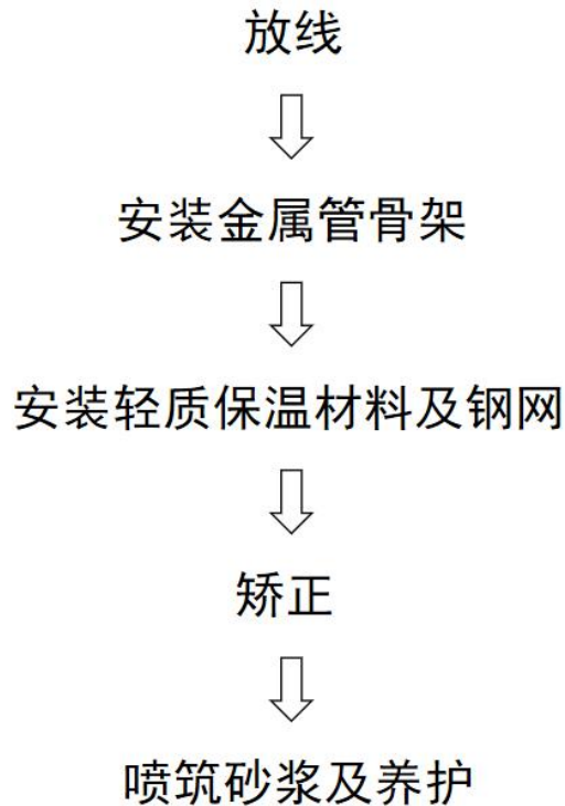
图 5 施工工艺流程
