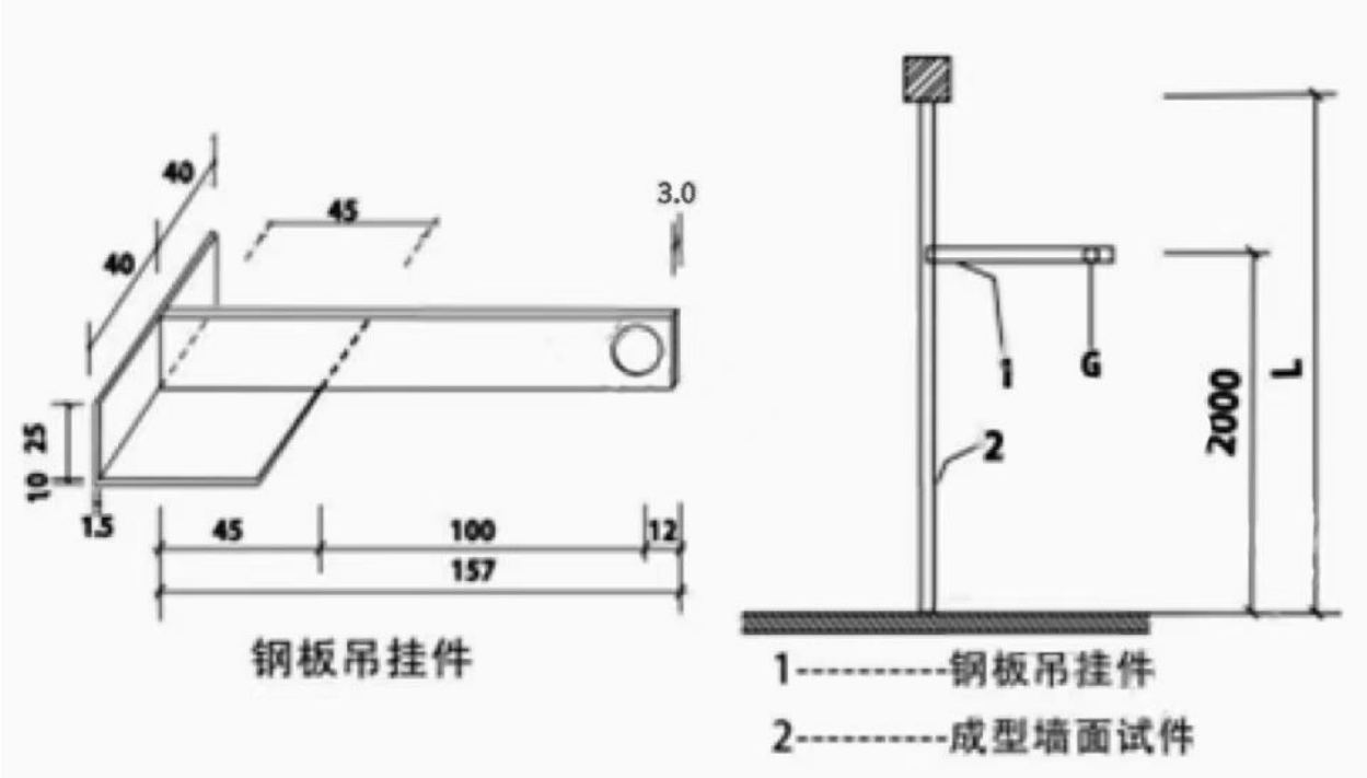
图 1 吊挂力试验装置
