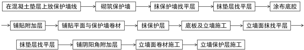
图 3 工艺流程图
