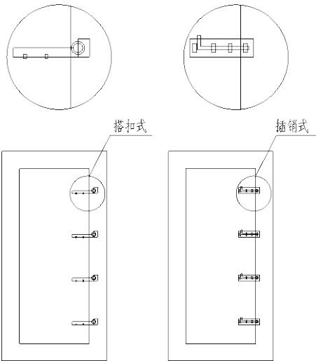
图5 搭扣式和插销式门板锁具示意
