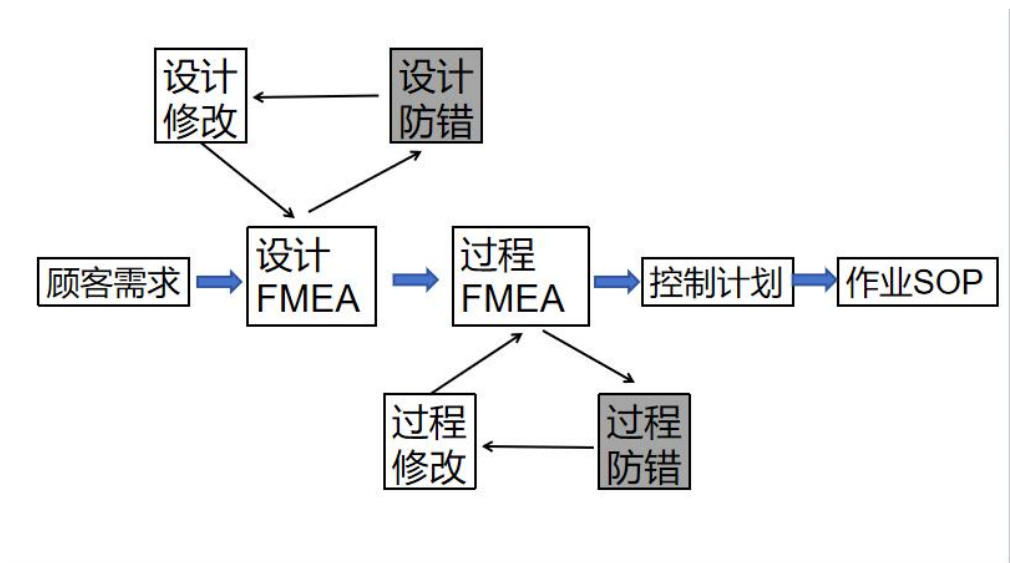
图 11 防错管理图
