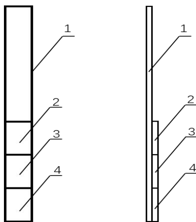
1. 底板，2. 吸油垫，3. 检测膜垫，4. 吸油垫
