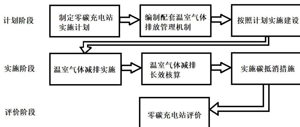
图1 光储充检一体化零碳充电站的实施流程
