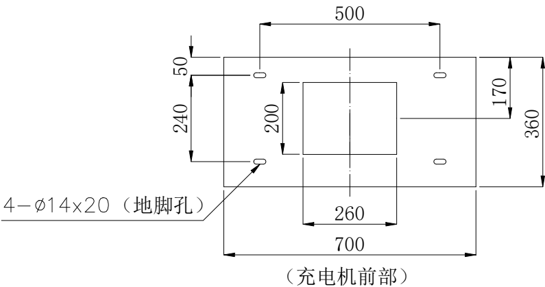
图 1 60/80kW 一体式充电机底座开孔尺寸（单位 mm）
