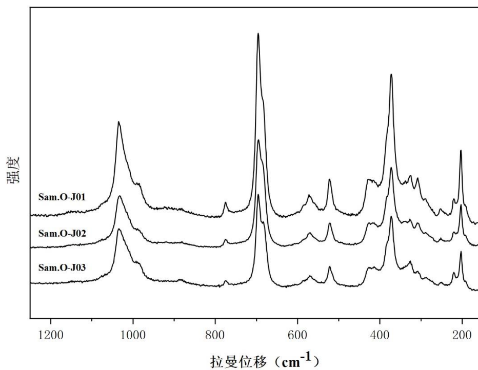
C.2 硬玉-绿辉石过渡玛雅绿翡翠拉曼光谱示例图
