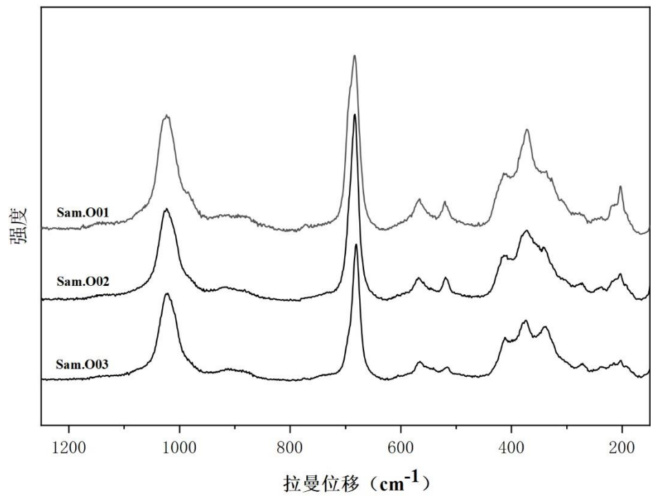
C.1 绿辉石为主玛雅绿翡翠拉曼光谱示例图
