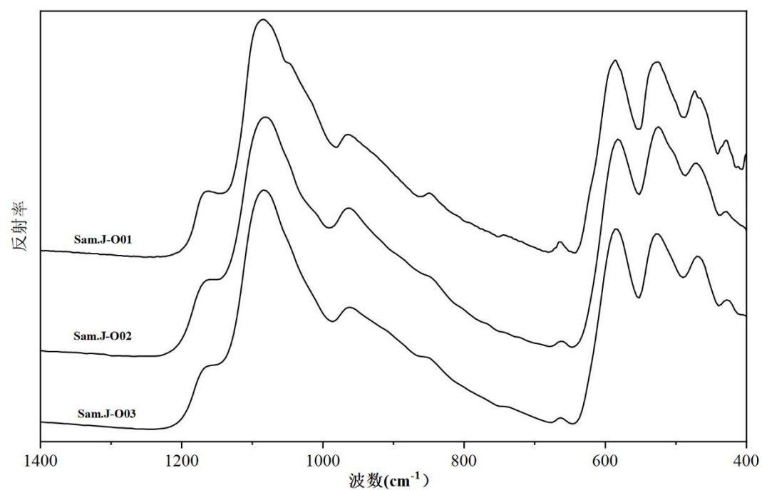
B.3 硬玉为主玛雅绿翡翠红外光谱示例图
