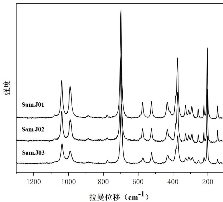
C.3 硬玉为主玛雅绿翡翠拉曼光谱示例图
