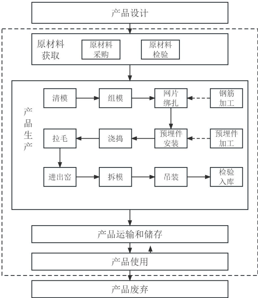
图 A.1 叠合板生命周期系统边界图
