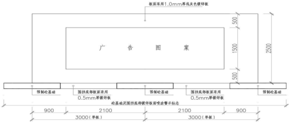
图1 围挡正立面图
