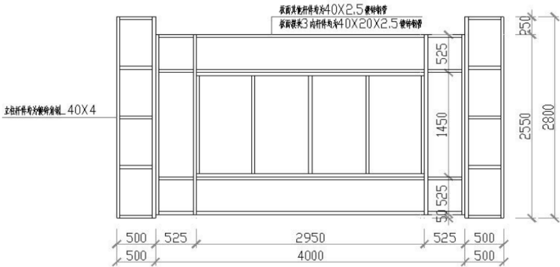
图2 围挡背立面图
