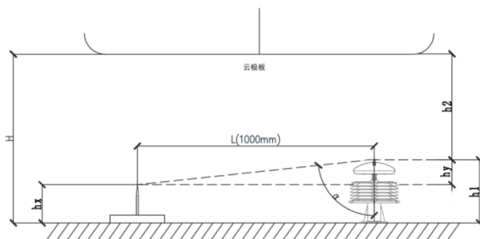
图1 试验装置示意图
