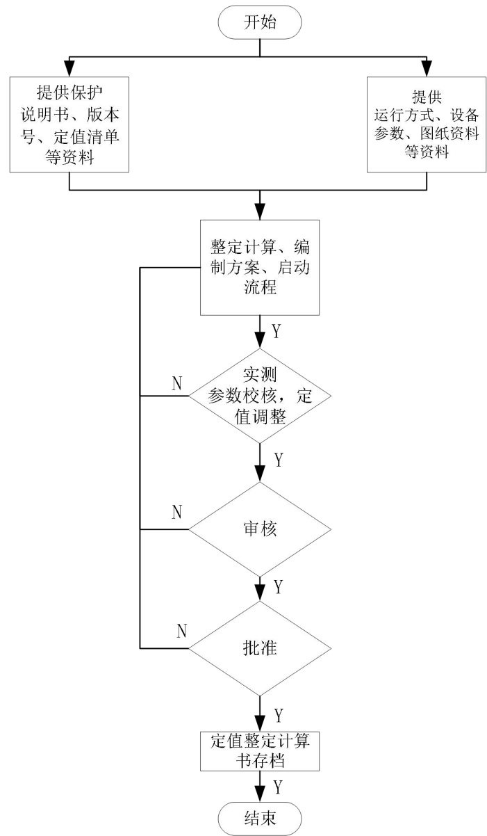
图 A.1 继电保护定值整定计算流程
