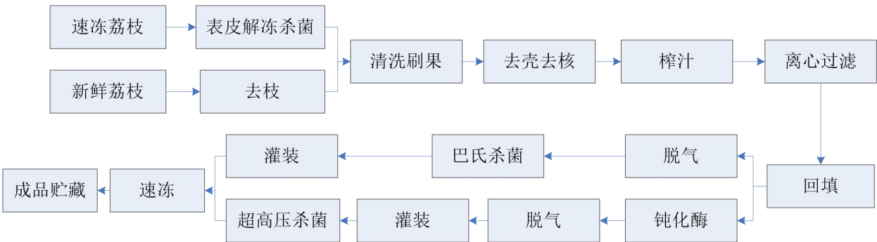
图1 工艺流程图
