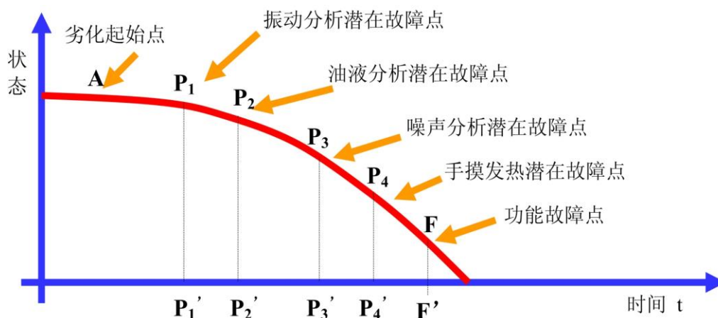
图 6 P-F 间隔时间与状态监测
