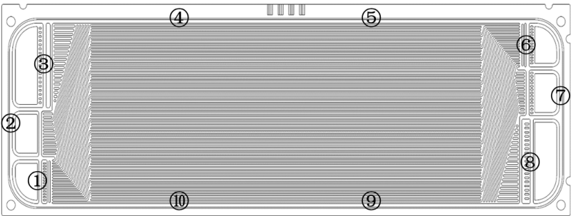
图4 密封槽深度测量点示意图
