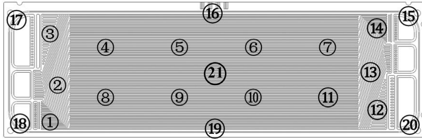
图3 极板厚度测量点示意图
