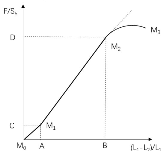
图7 极板应力-应变示意图
