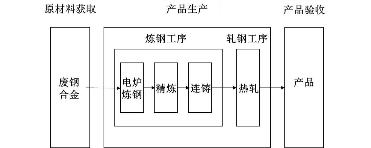
图 B.2 输电线路铁塔用热轧角钢生命周期系统边界示意图（电炉生产工艺）
