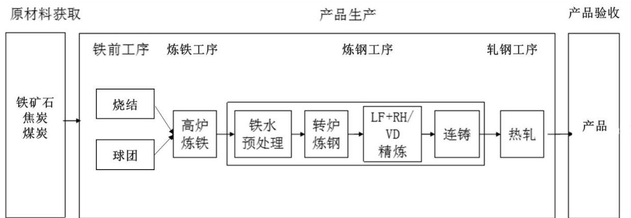
图 B.1 输电线路铁塔用热轧角钢生命周期系统边界示意图（高炉-转炉生产工艺）
