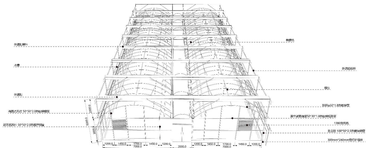
图 A.3 双膜双网连栋温室 II 型
