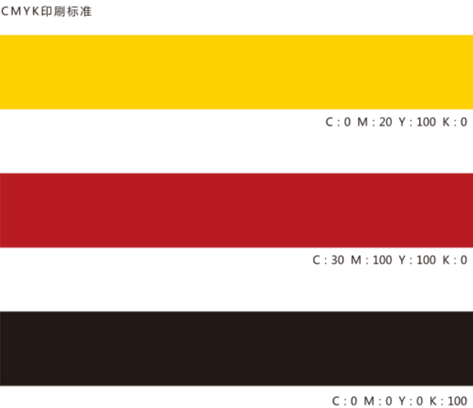
图4 标准色值
