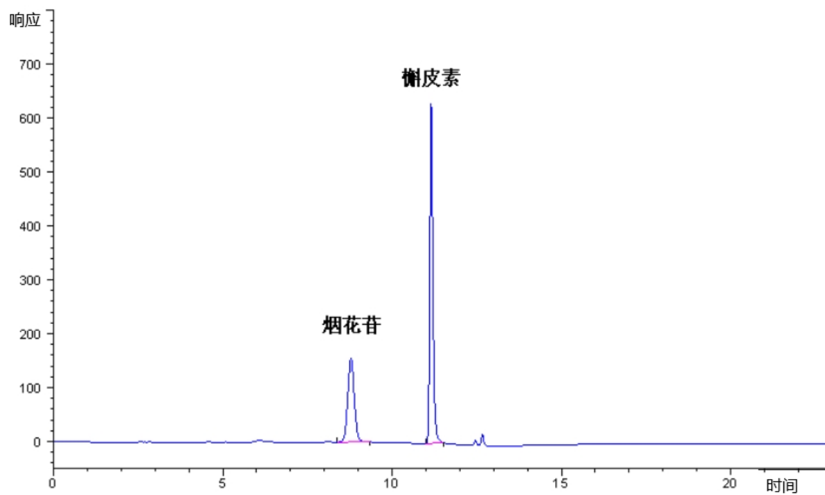
图 A.1 烟花苷、槲皮素的色谱图
