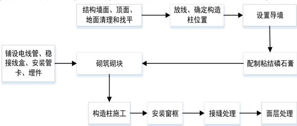
图 4 磷石膏砌块施工工序
