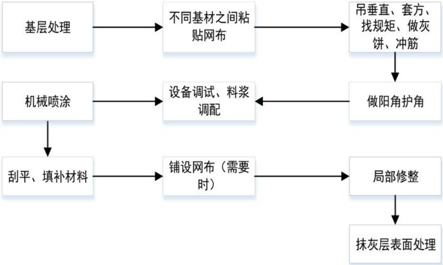
图 2 机喷抹灰施工工序
