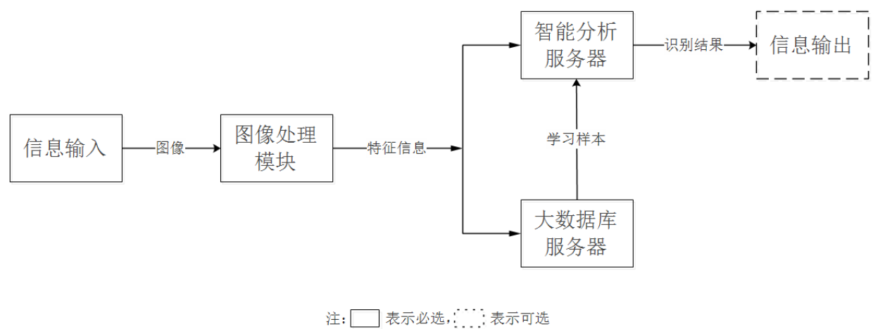
图3 数据分析子系统组成及工作流程
