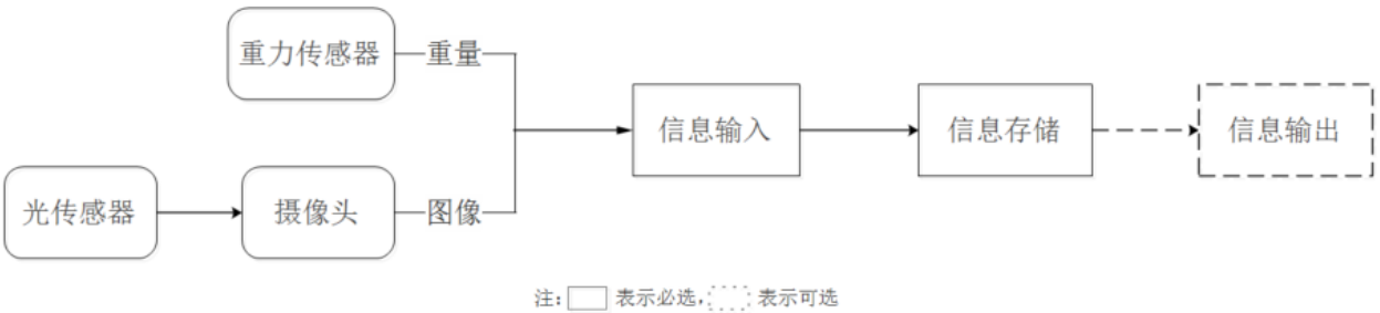
图2 数据采集子系统组成及工作流程
