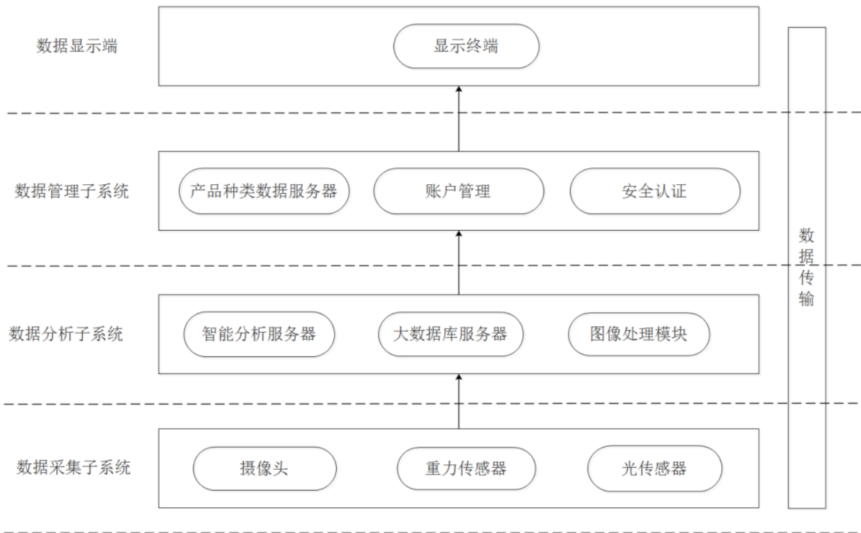
图1 鱼类种类智能识别管理系统架构
