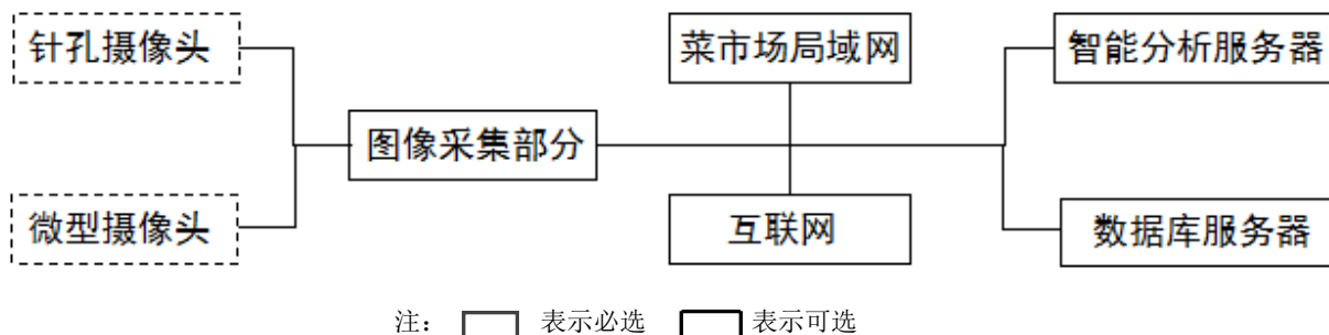
图4.2 智能电子秤子系统组成架构图
