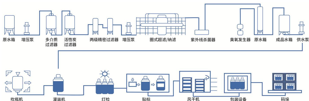
图 1 生产工艺流程图
